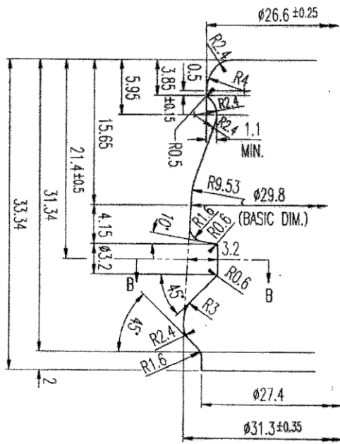
A-A SECTION (S=3/1)
