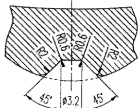
B-B SECTION (S=3/1)
