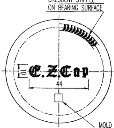
B-B SECTION (S=3/1)
