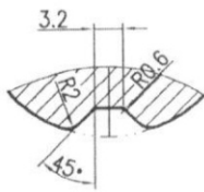
A--A 2:1
